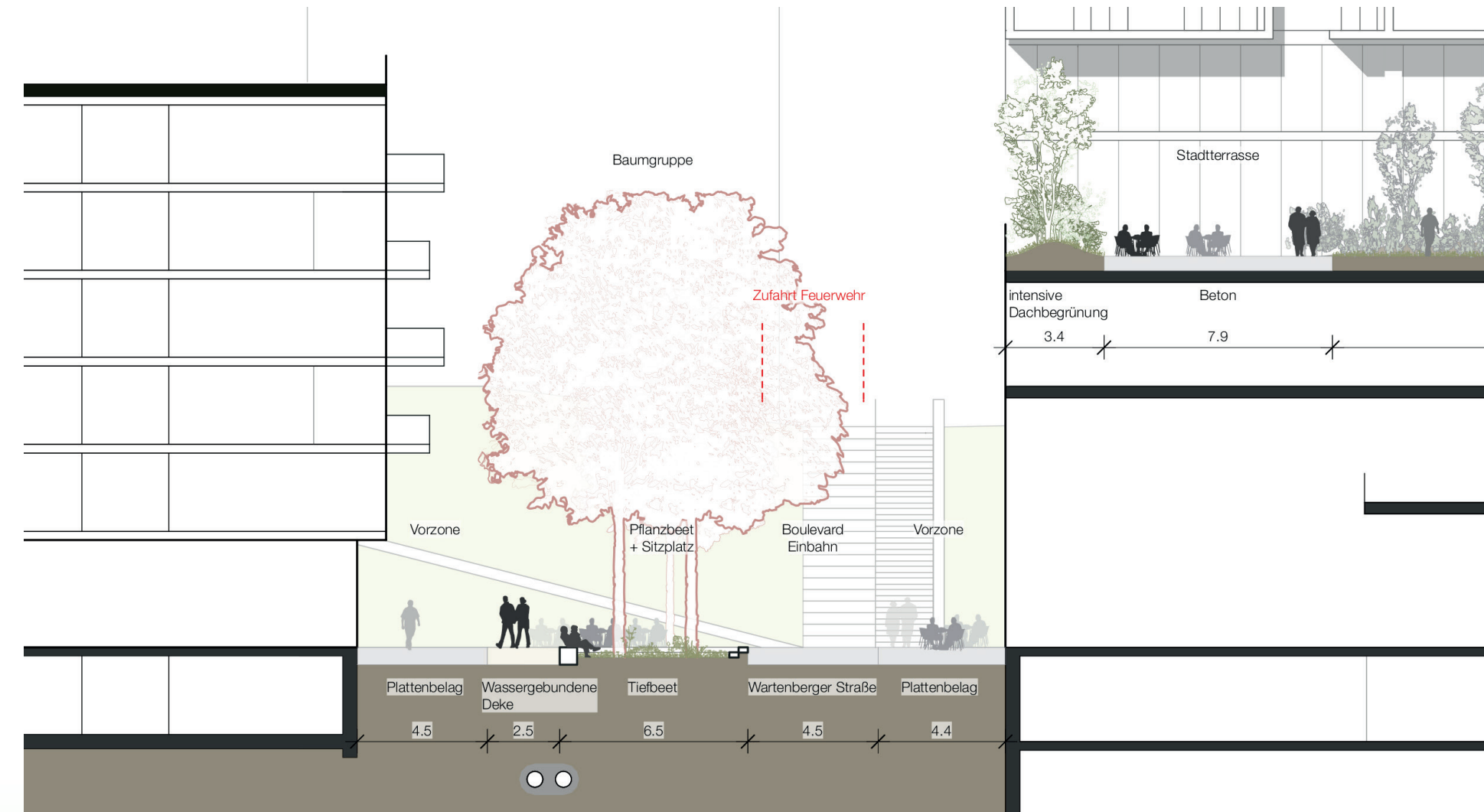
BOULEVARD SCHNITT
