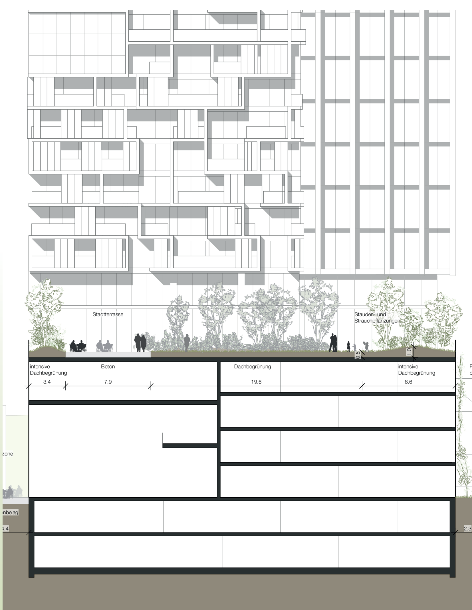
SCHNITT SOCKELGESCHOSS MIT DACHGARTEN
