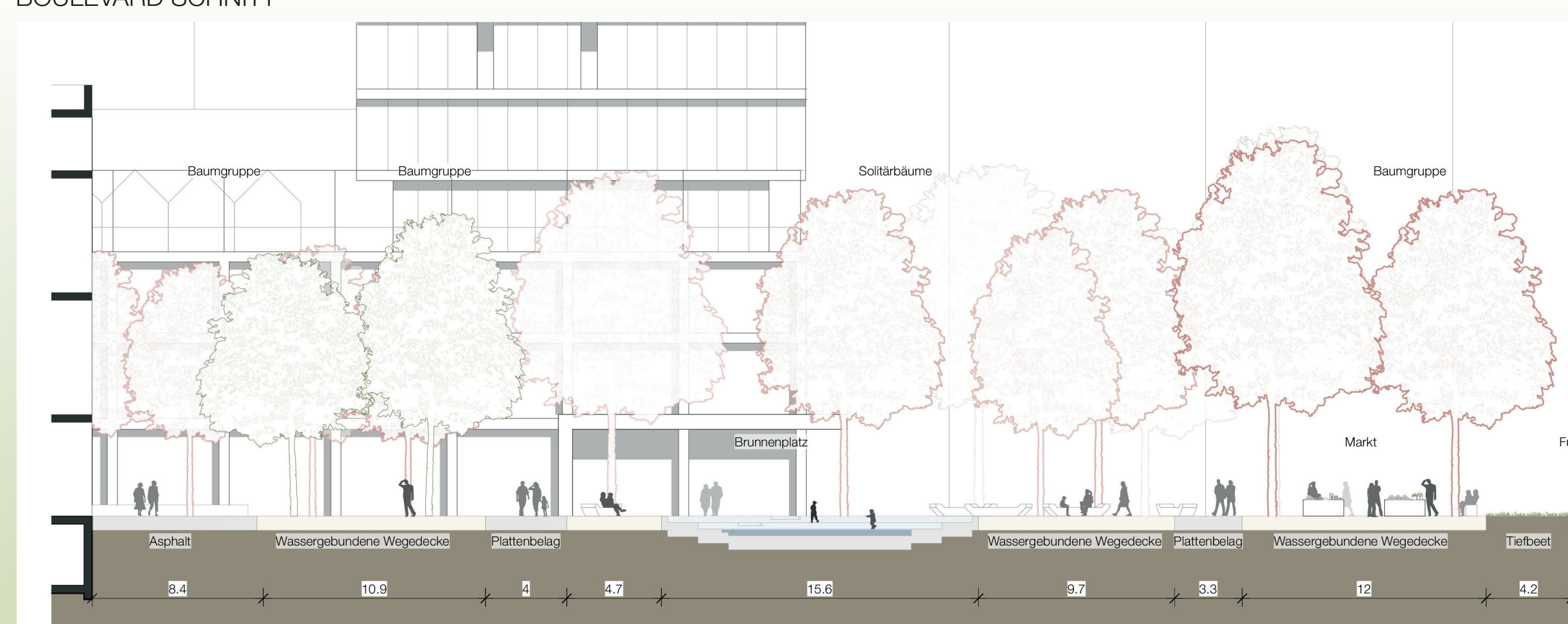
BRUNNENPLATZ SCHNITT
